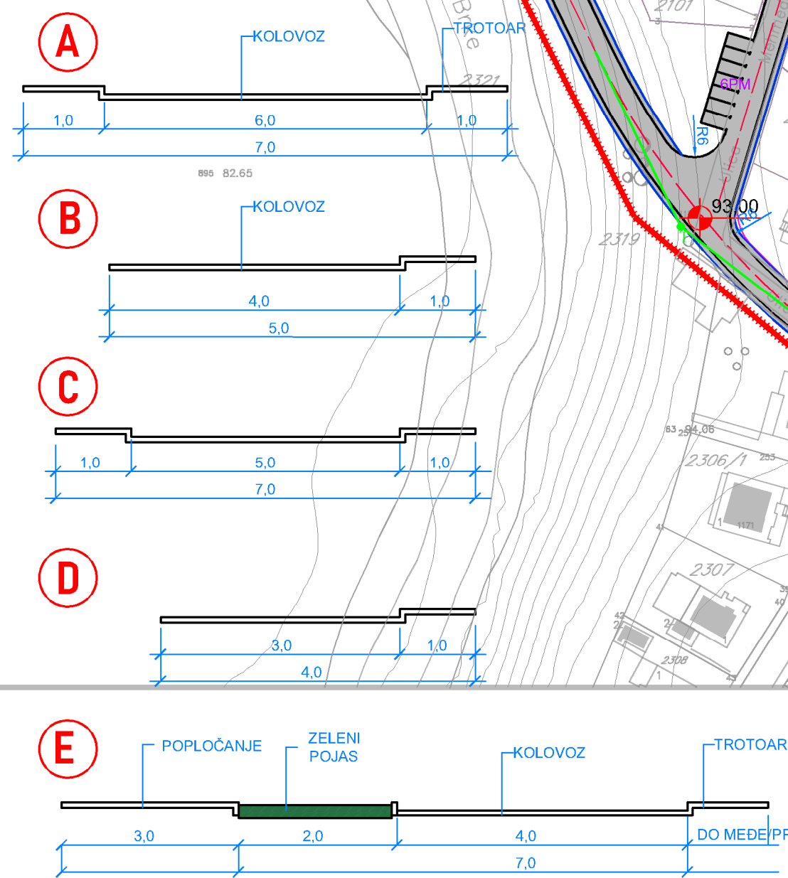
PROFILI SAOBRAĆAJNICA
